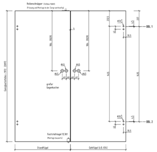
Bohrungsvariante 5, 2-flg.
